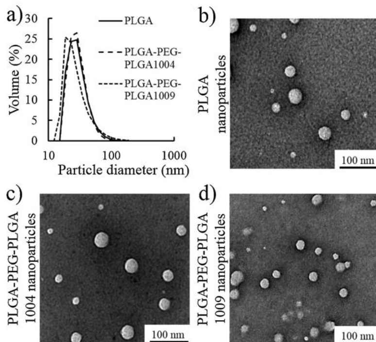
図 : (a) CsA を搭載した PLGA、PLGA-PEG-PLGA1004、および PLGA-PEG-PLGA1009 ナノ粒子の粒子サイズ分布 (n = 3)。100 kV の加速電圧で撮影した CsA 搭載 PLGA (b)、PLGA-PEG-PLGA1004 (c)、および PLGA-PEG-PLGA1009 ナノ粒子 (d) の TEM 画像 (倍率: 10,000 倍)。
